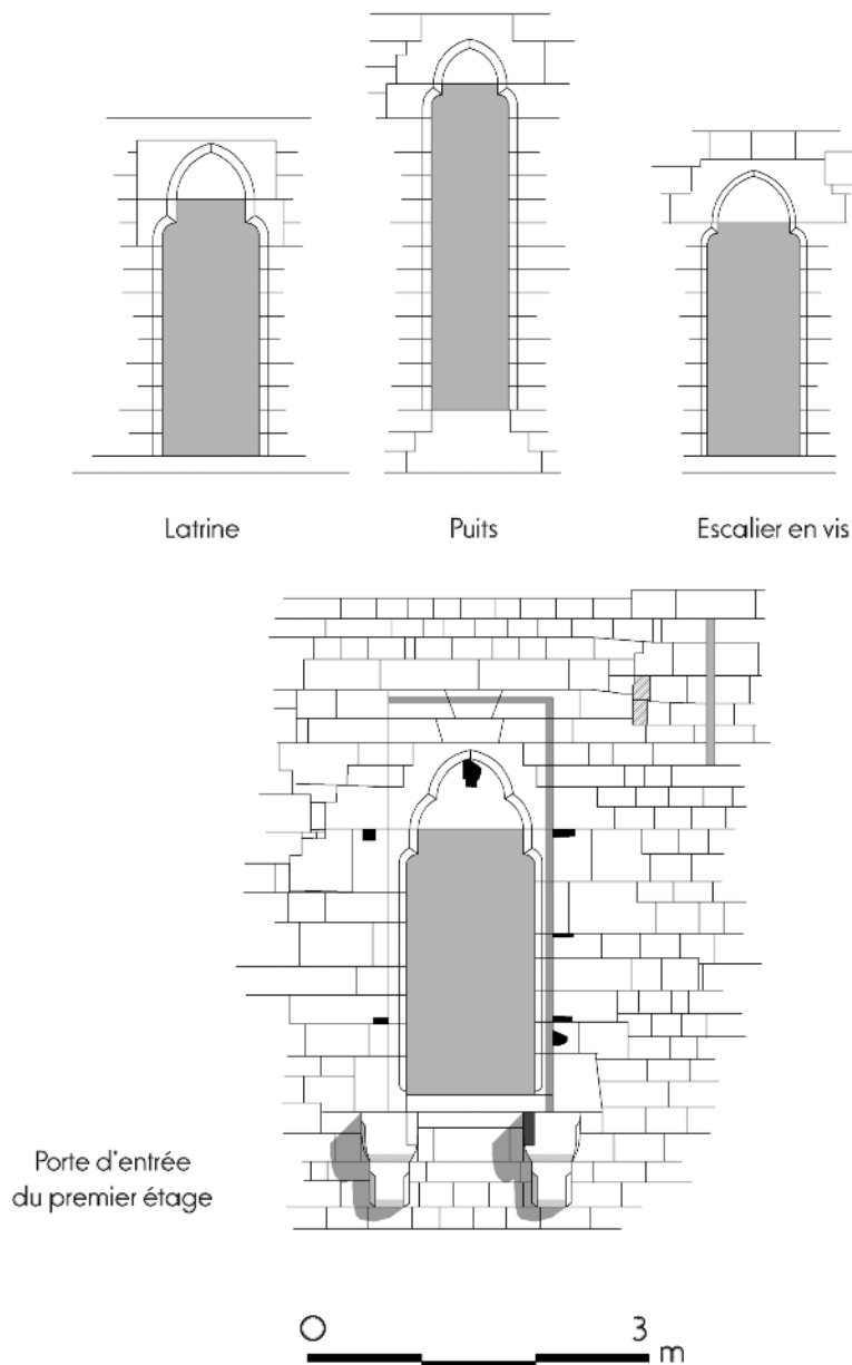
Fig. 13 - Vernon, élévations des portes de la tour maîtresse (dessin J. Mesqui). En haut, portes intérieures du rez-de-chaussée. En bas, porte extérieure du premier étage de la tour, dans son état actuel.
